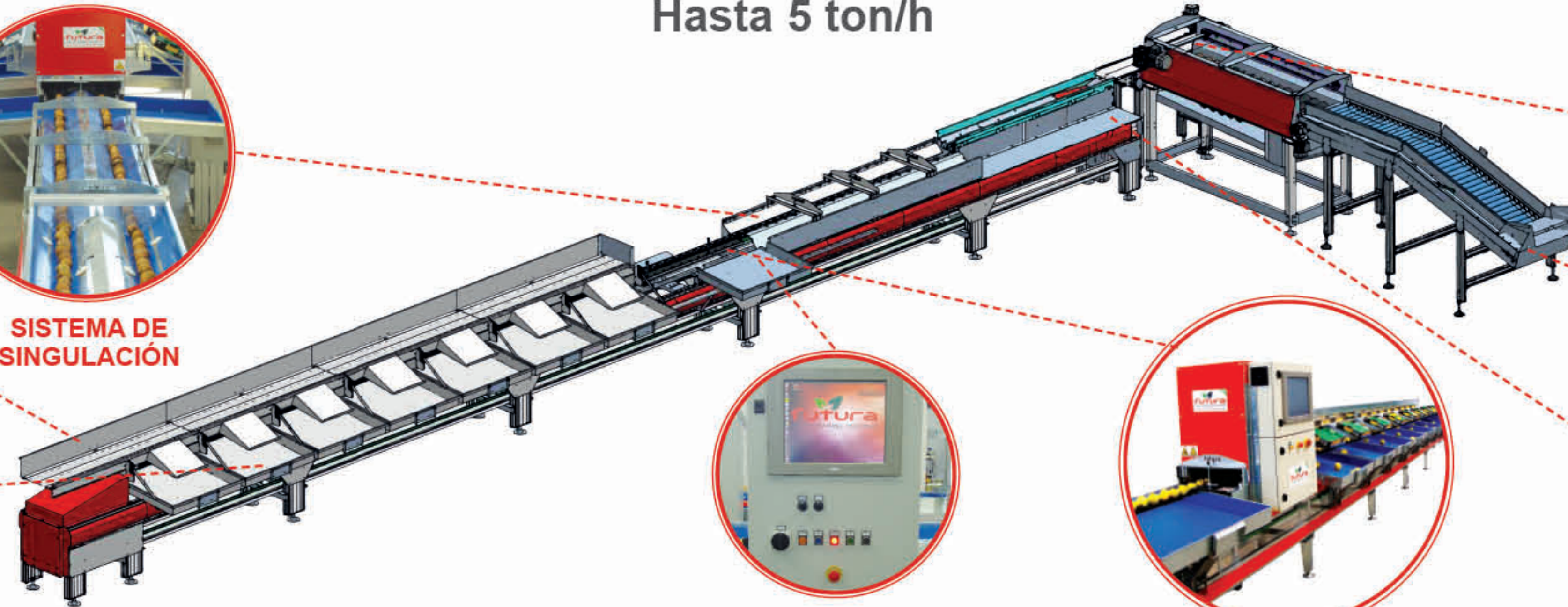
PANEL DE CONTROL GENERAL CON CONEXIÓN REMOTA POR TELEASISTENCIA
